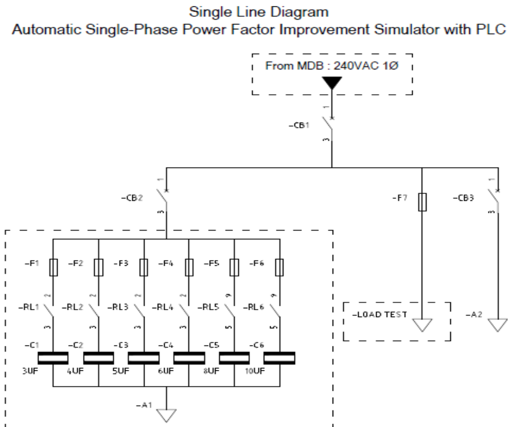
ภาพที่ 1 แสดงผังการวงจรการต่อคาปาซิเตอร์เข้ากับระบบเพื่อปรับปรุงเพาเวอร์แฟคเตอร์ของโหลด
